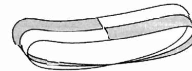
Möbius band
